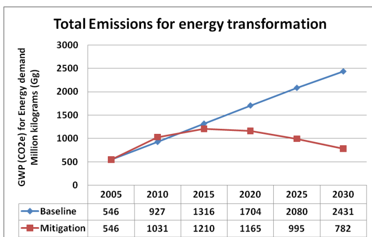
Figure 17a: Emissions totales provenant de la transformation énergétique
