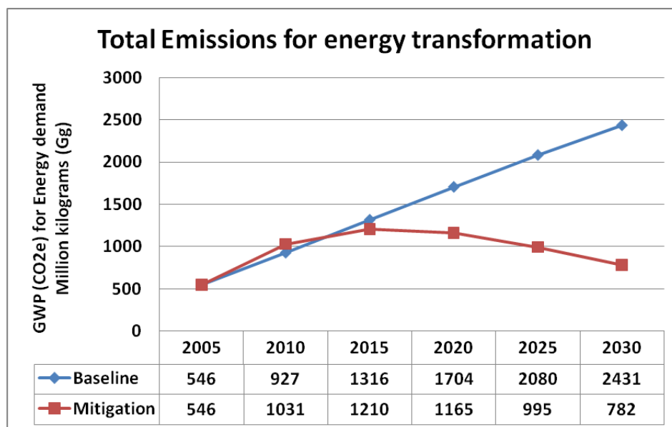
Figure 19a: Emissions totales provenant de la transformation énergétique
