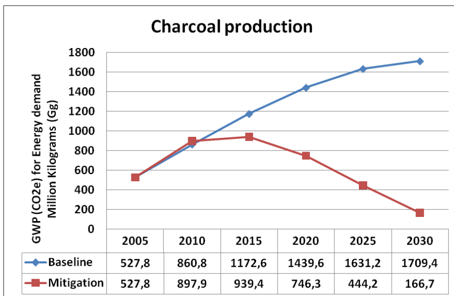
Figure 19c: Emissions provenant de la production du charbon
