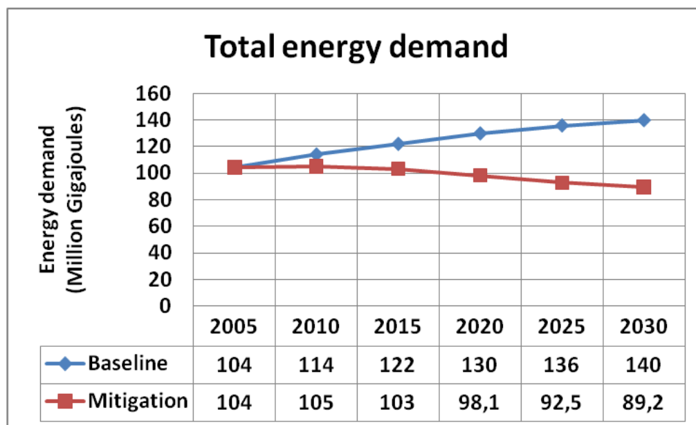
Figure17a: Demande énergétique totale
