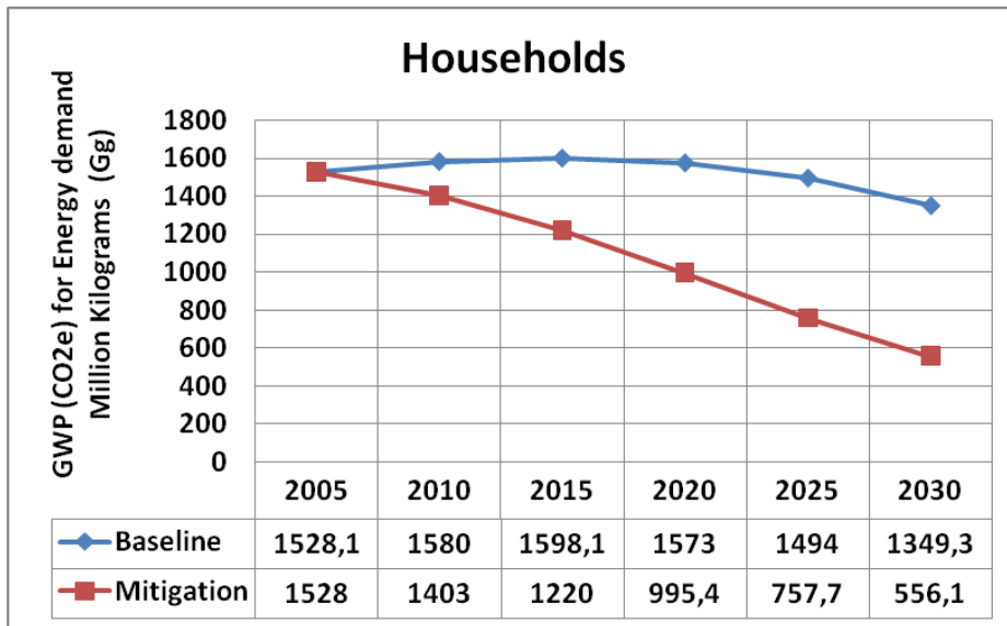
Figure18b: Emissions provenant de la demande énergétique/Ménages
