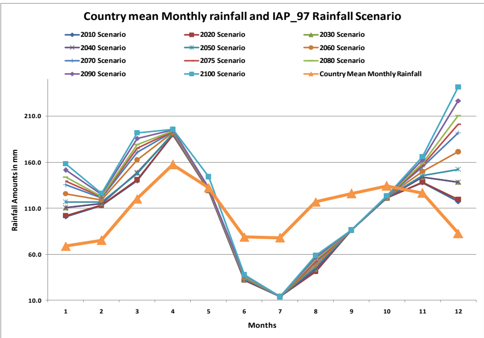
Figure 25b: Scénarios des pluies, IAP_97
