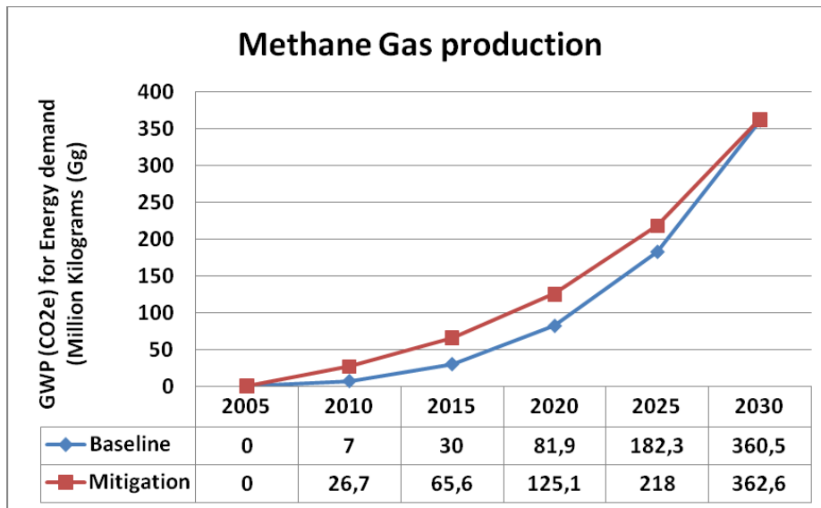
Figure19d: Emissions provenant de la production du gaz méthane
