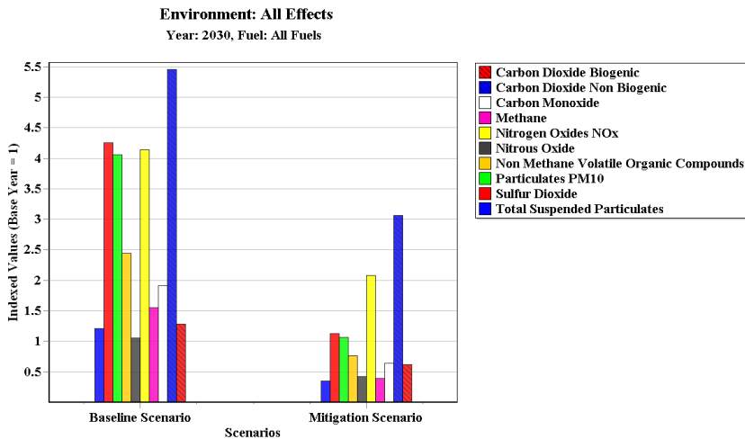
Figure19: Effet des options proposées sur l'environnement
