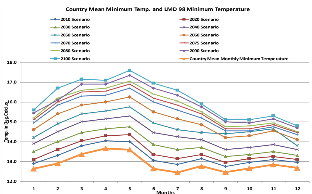
Figure 22c : Température minimum projetée du modèle LMD_98
