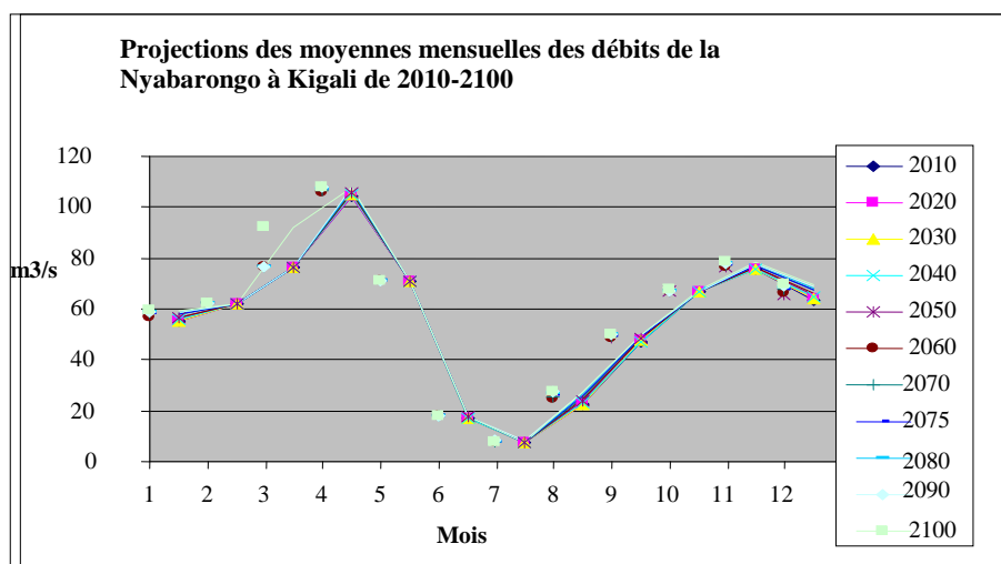
Figure 28: Projections des moyennes mensuelles des débits de la Nyabarongo à Kigali (2010-2100)
