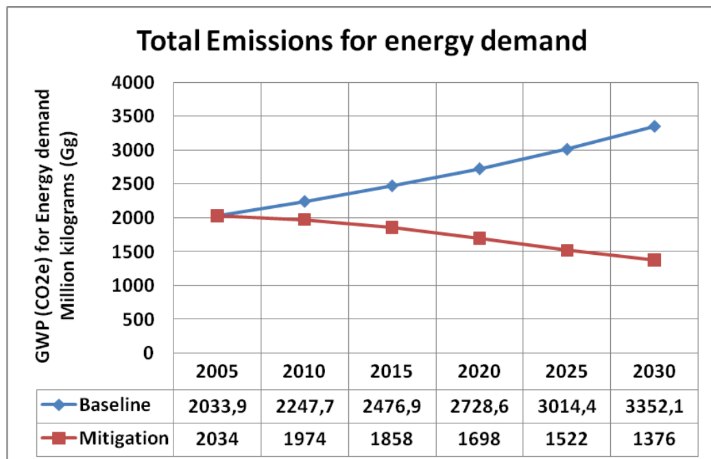
Figure18a: Total des émissions provenant de la demande énergétique
