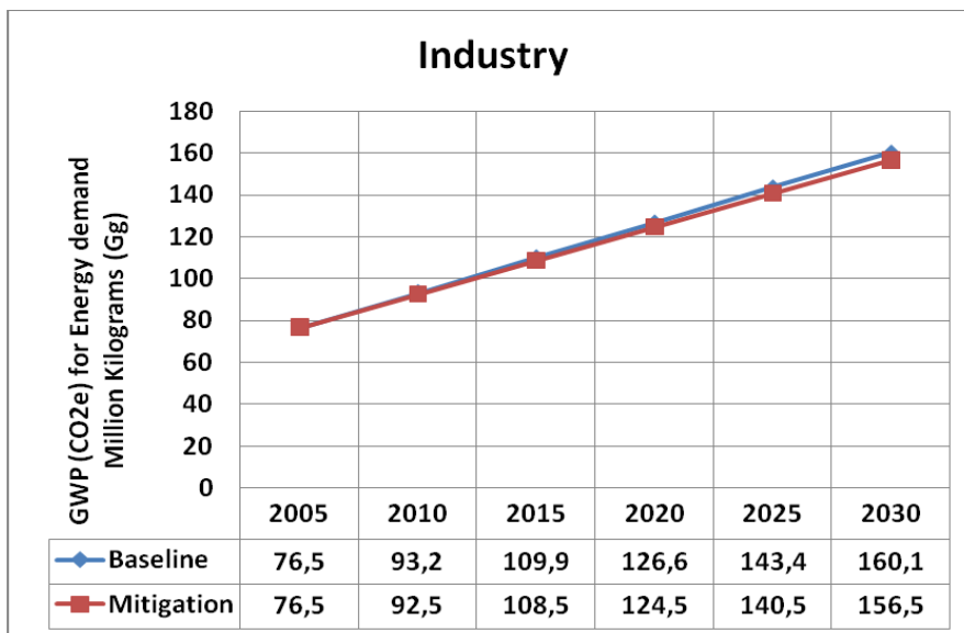
Figure18c: Emissions provenant de la demande énergétique/Industrie
