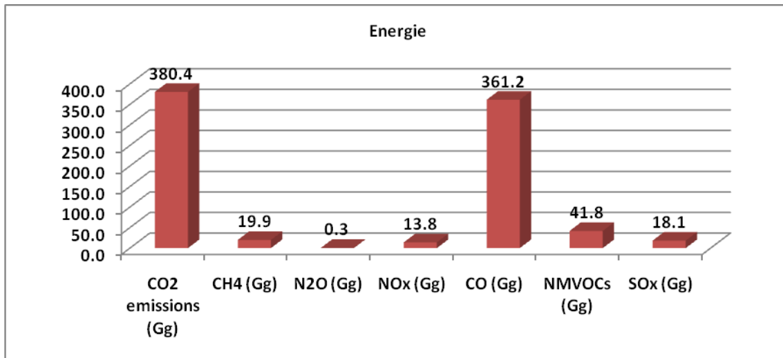
Figure 9: Emissions totales de GES pour le secteur de l'énergie en 2005
