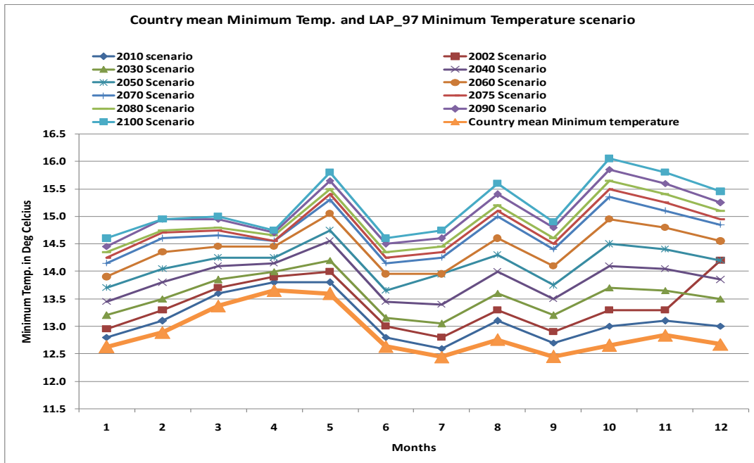
Figure 22b: Température minimum projetée du modèle IAP_97
