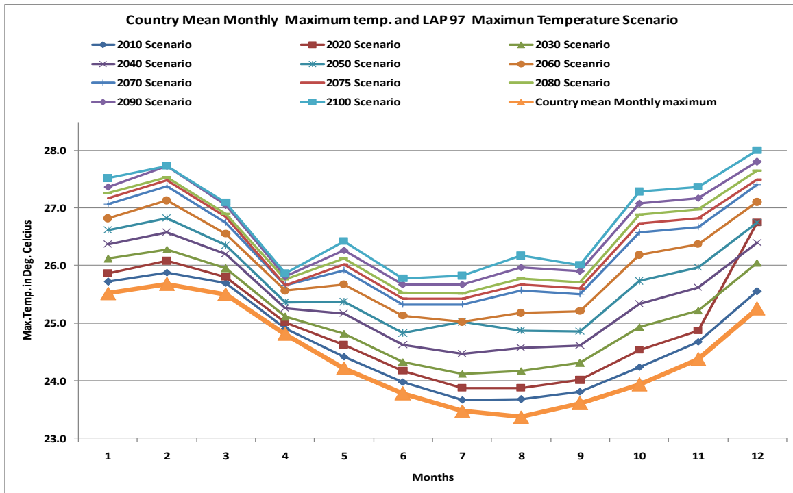
Figure 24b: Température maximum projetée du modèle IAP_97
