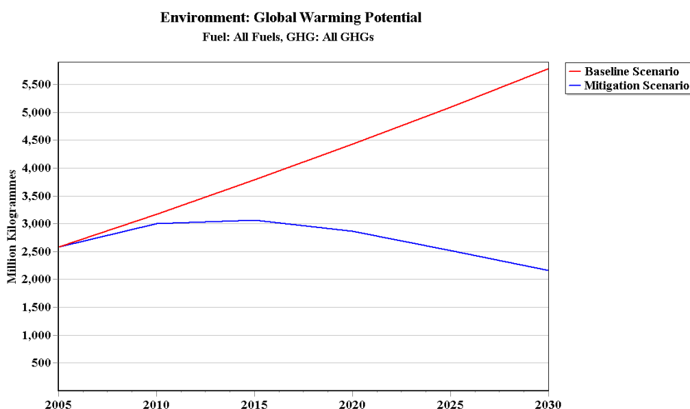
Figure 20: Evolution des émissions totales réduites
