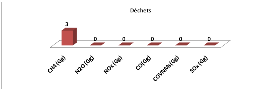
Figure 13: Emissions de GES pour le secteur des déchets en 2005
