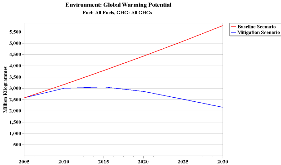
Figure18: Evolution des émissions totales réduites
