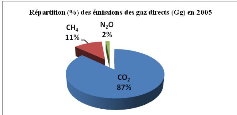
Figure 8: Répartition des émissions des gaz directs (%) en 2005
