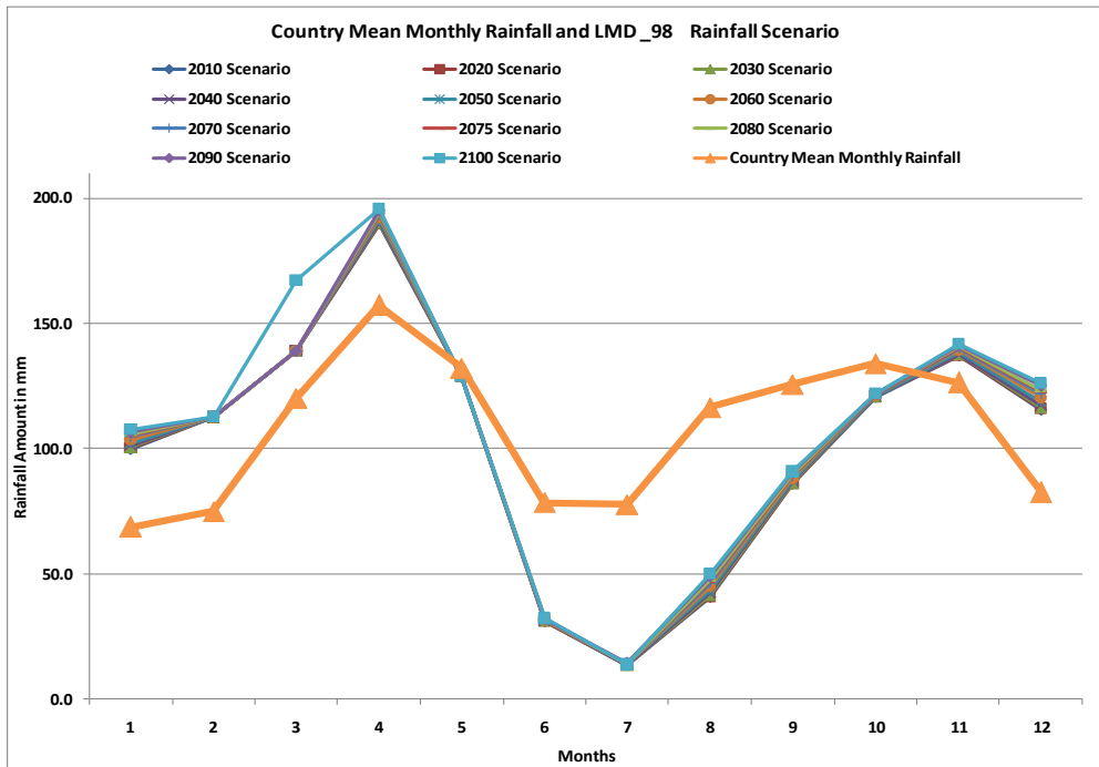
Figure 25c: Scénario des pluies, LMD_98
