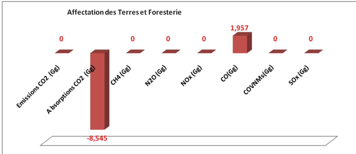
Figure 12: Emissions de GES pour le secteur de l'UTCATF en 2005
