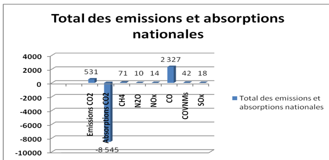
Figure 7: Emissions de GES en 2005 en Gg
