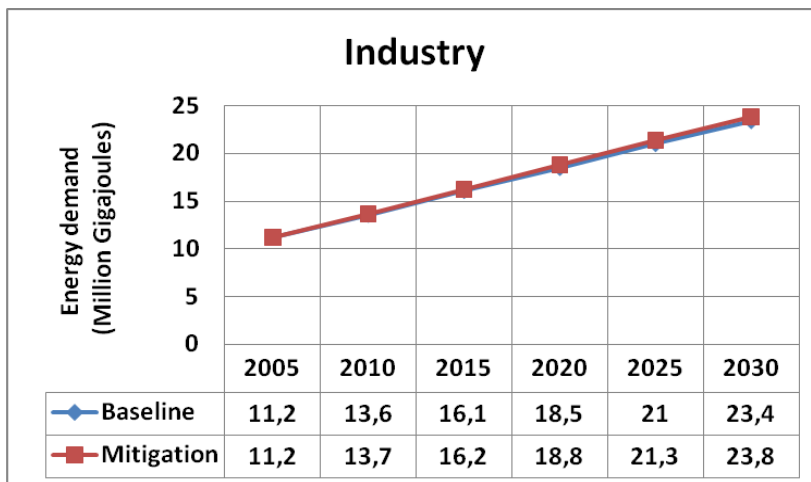
Figure 17c : Demande énergétique des industries
