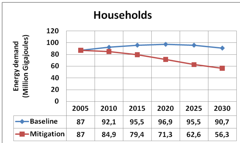
Figure 17b : Demande énergétique des ménages
