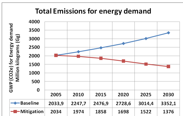
Figure16a: Total des émissions pour la demande énergétique
